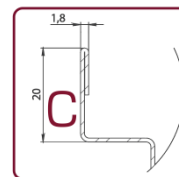
Конвектор С БЕЗ ДЕКОРАТИВНОЇ РАМКИ
