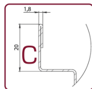
конвектор С без декоративної рамки
