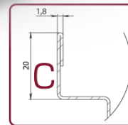
конвектор C без декоративної рамки
